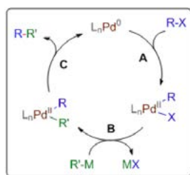
Création d'une liaison carbone-carbone catalysée par un complexe organométallique à base de palladium
