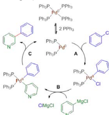
Création d'une liaison carbone-carbone catalysée par un complexe organométallique à base de palladium
