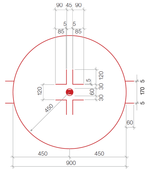
Toutes les dimensions en cm
