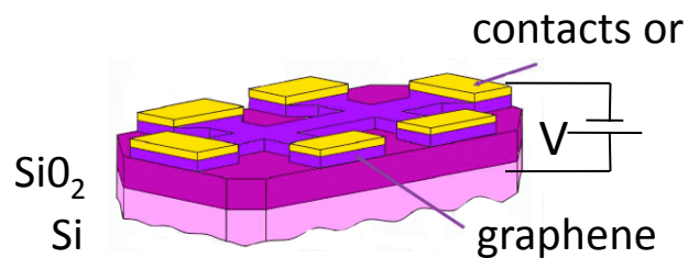
Dispositif de mesure de conductivité
